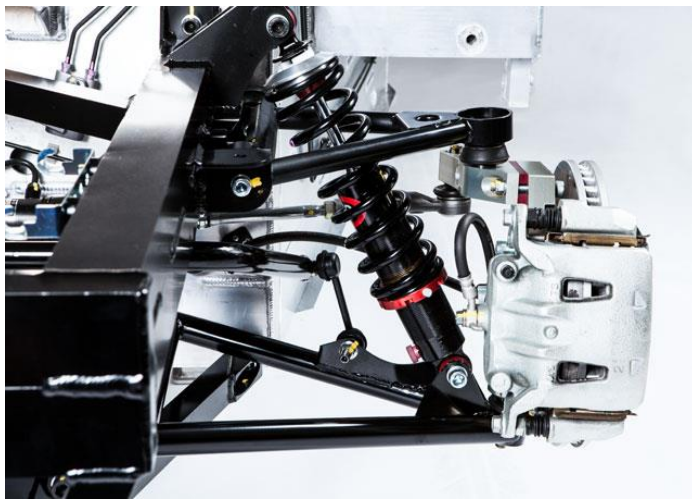
フロントサスペンション
